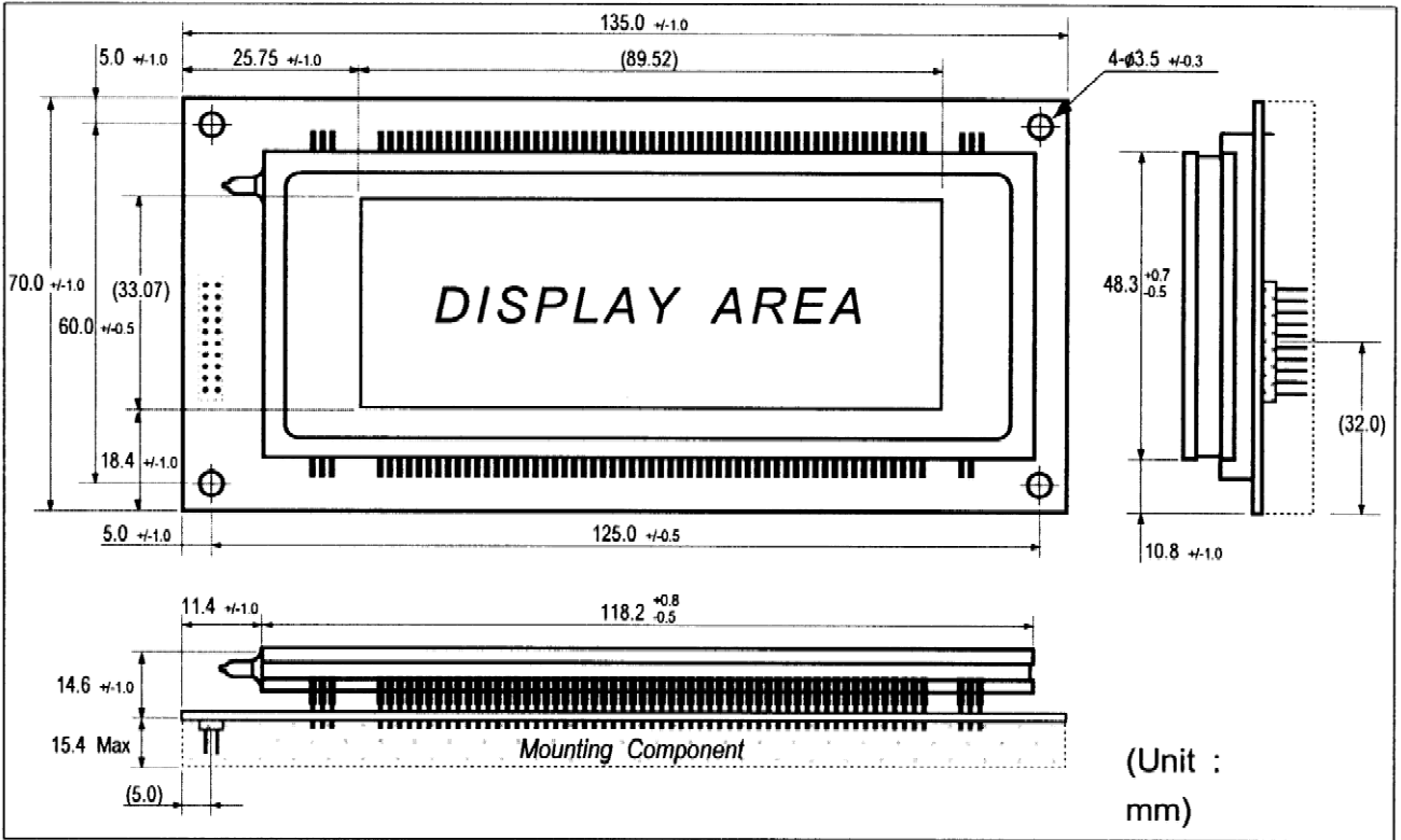
Fig-3. Outer Dimensions
